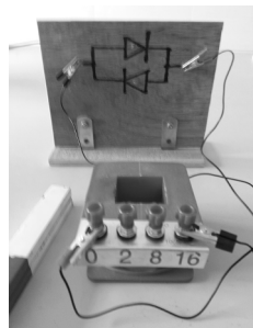
图3 自制验证楞次定律的实验装置
